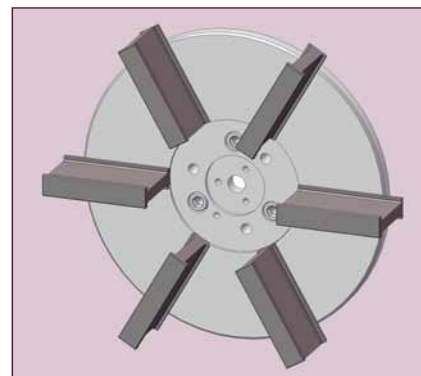
Wirnik jednotarczowy firmy AGTOS z 6 łopatkami turbinowymi.
