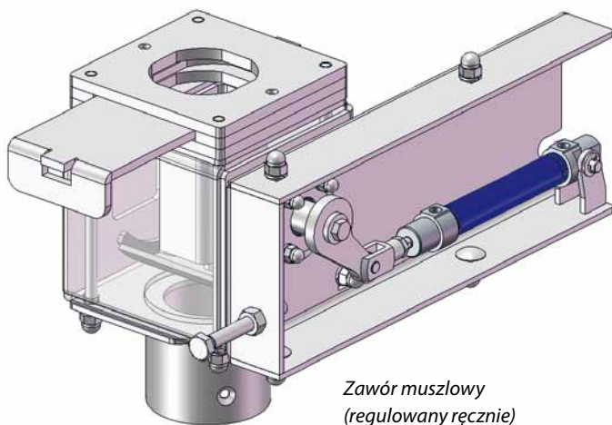
Zawór muszlowy dozujący (sterowany elektronicznie poprzez szafę sterowniczą)
