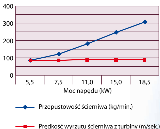
Przepustowość ścierniwa w turbinach TA 3.6, Ø wirnik 380 mm
