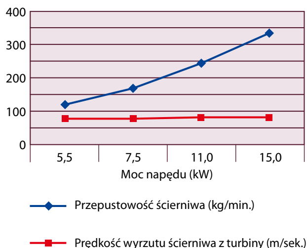
Przepustowość ścierniwa w turbinach TA 3.6, Ø wirnik 330 mm
