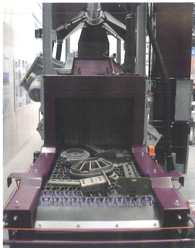
Części odlewane przed oczyszczarką strumieniową z taśmą z plecionego drutu stalowego firmy AGTOS.
